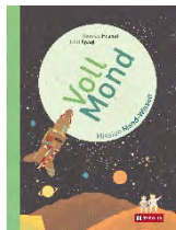
Moon
